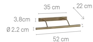
RÉFLECTEUR TABLEAUX 9004 BR G9 4x 4W LED max Réflecteur pivotant à 360°
