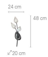
APPLIQUE SPARTE 3L SG A210 G9 3x 5W LED maxi
