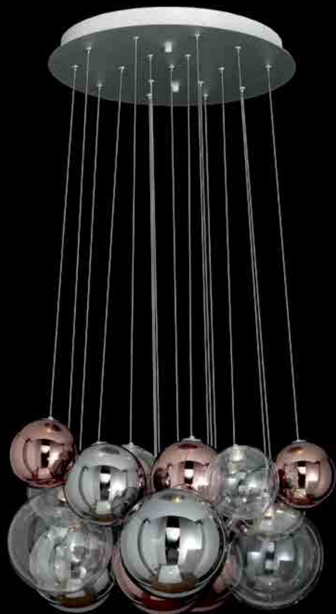
LCS 040/18 Arg/C Ø 60 cm - H. max 200 cm Ø delle sfere 120/140/180 mm Led 18x2W
